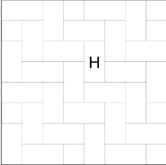
Pattern YKT.05 - Herringbone
