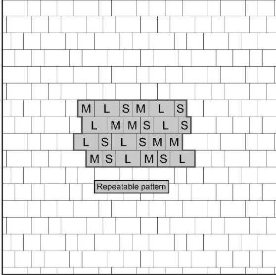
Pattern LUG.05 - 3 Size Stretcher - P & L*
