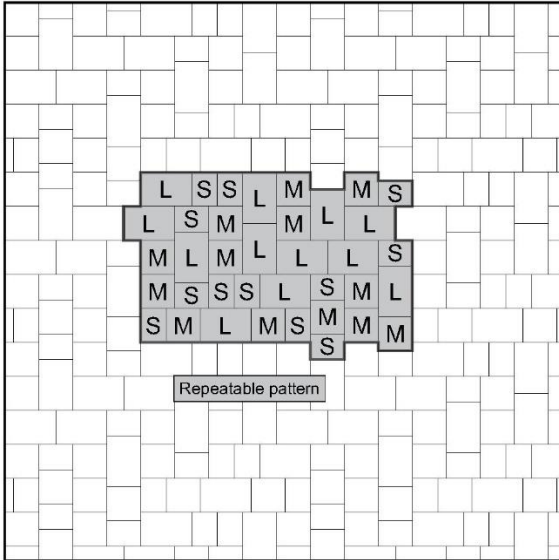
Pattern LUG.09 - 3 Size Stretcher - P & L
