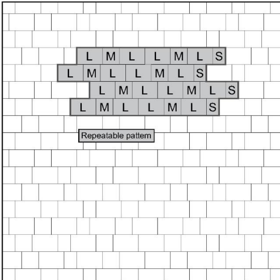
Pattern LUG.07 - 3 Size Stretcher - P & L*
