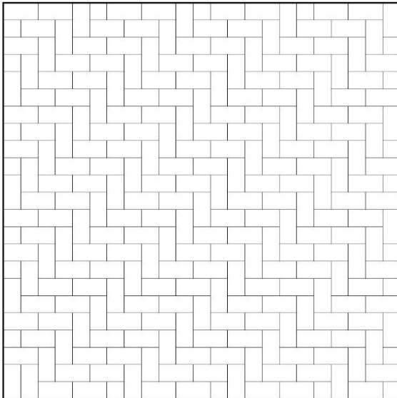
Pattern ONP.07 - Herringbone 2:1 - P & L
